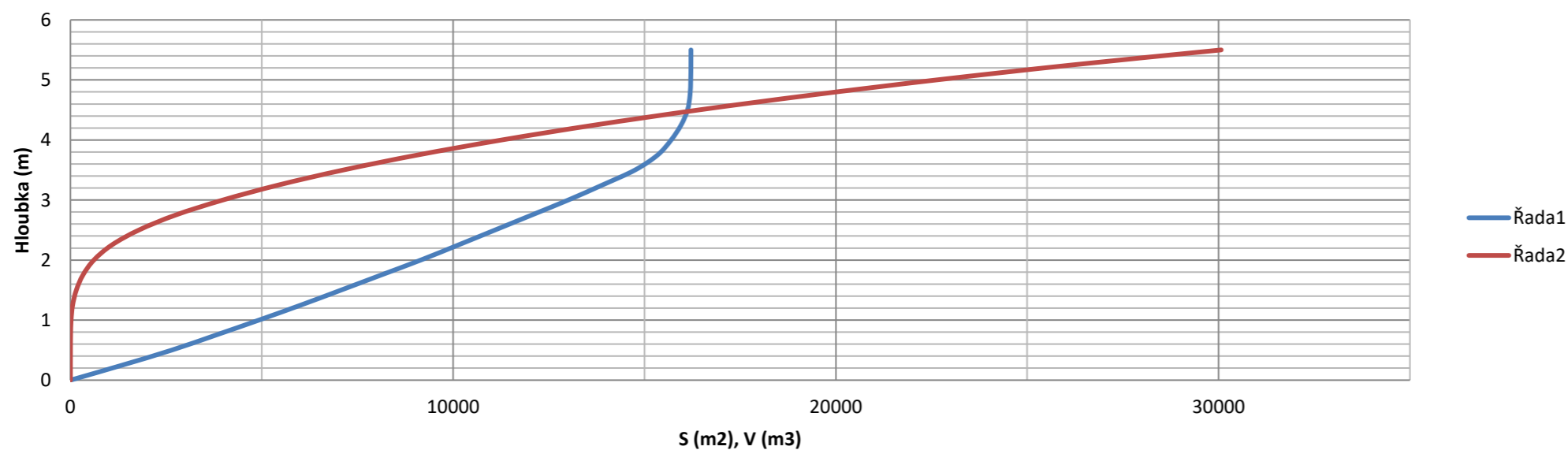
Batygrafické křivky
