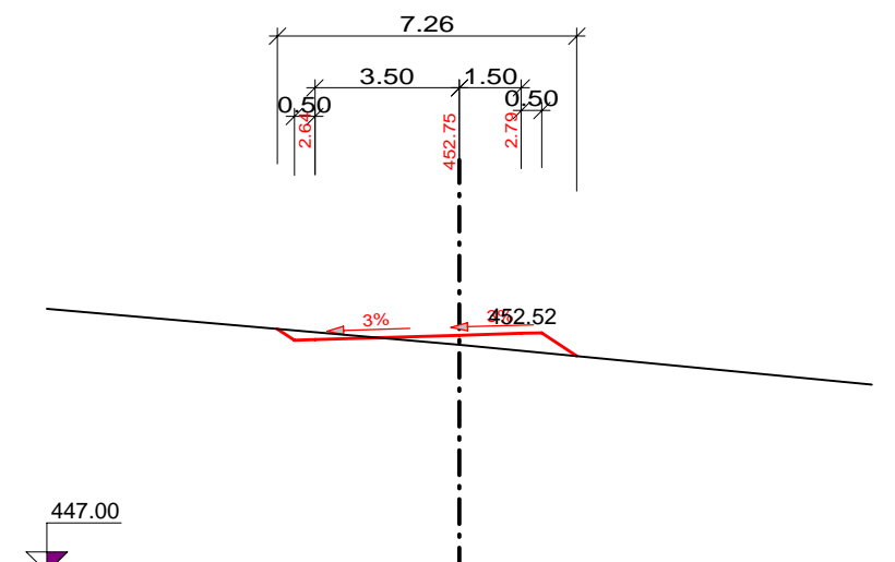
114 - KM 1.13000 výhybna NV3
