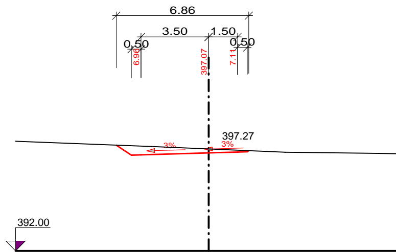
41 - KM 0.40000 výhybna NV1
