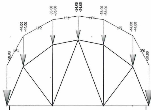
Obrázek 18 – Zatížení podpůrné konstrukce při poklesu zdiva
