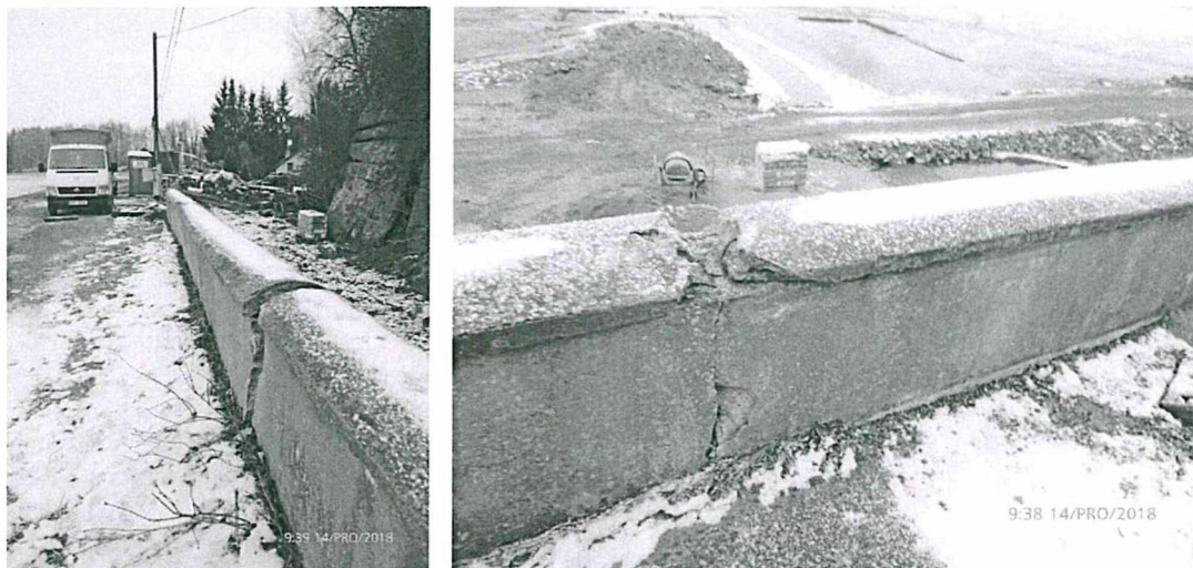
Obrázek 11 – Poškození vozovky a parapetní zdi trhlinami a vykloněním zdi v oblasti mostu
