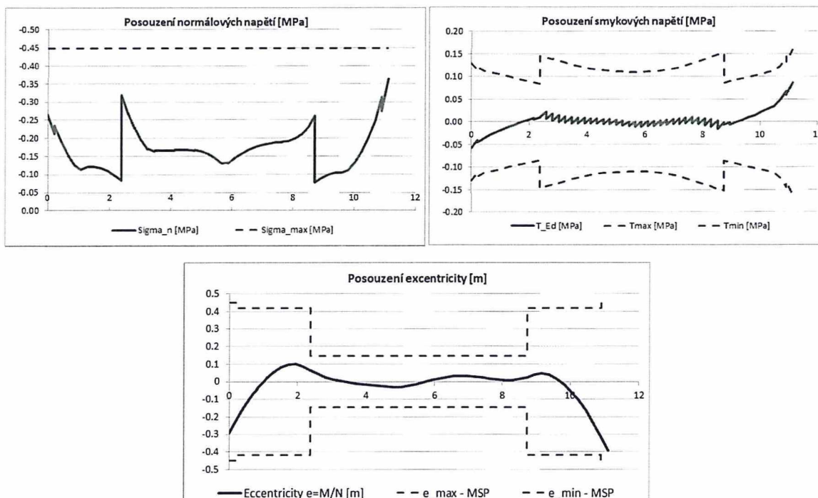
Obrázek 16 – Výstupy ověření konstrukce v mezním stavu použitelnosti => plná zatížitelnost
