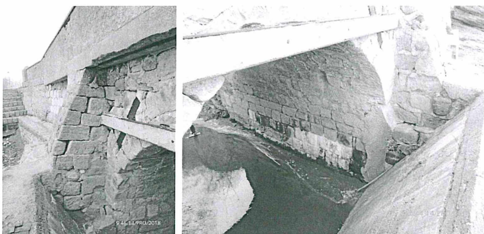
Obrázek 6 – Rozvolnění zdiva zesilujících pilířů na návodní straně mostu, stav zesílení klenby
