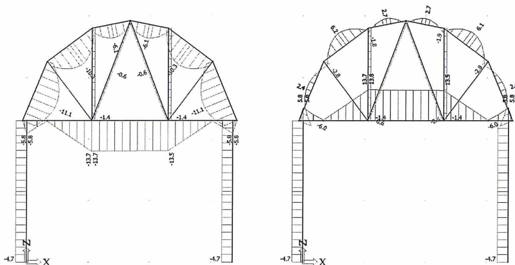
Obrázek 19 – Normálová napětí v podpůrné konstrukci v MSÚ \sigma_{\max} < 14 \text{ MPa} \Rightarrow \text{Vyhovuje}
