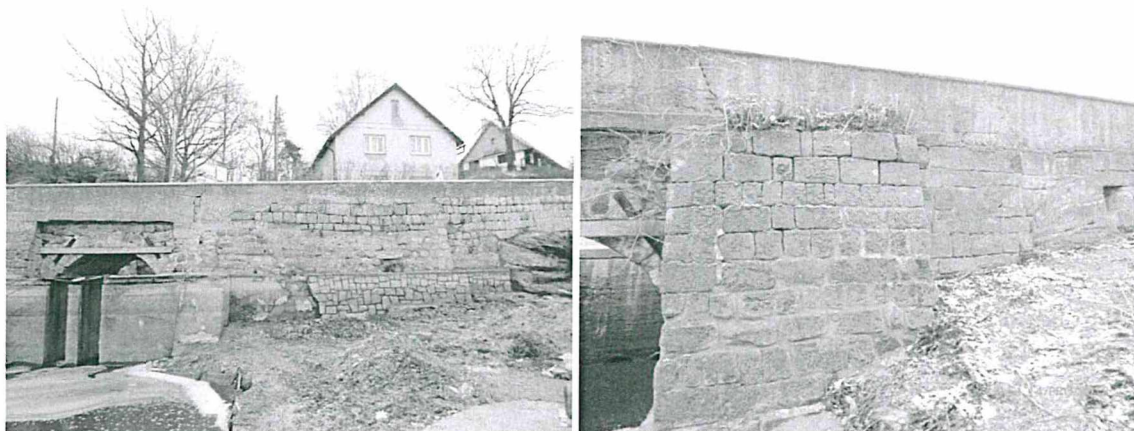
Obrázek 5 – Stav navazujících křídel (vlevo návodní strana, vpravo povodní strana)
