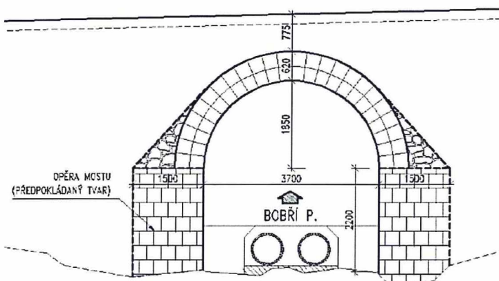
Obrázek 12 – Model konstrukce pro ověření odolnosti
