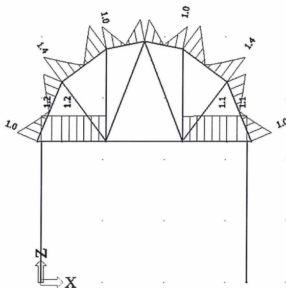
Obrázek 20 – Smyková napětí v podpůrné konstrukci v MSÚ \tau_{\max} < 3,0 \text{ MPa} \Rightarrow \text{Vyhovuje}
