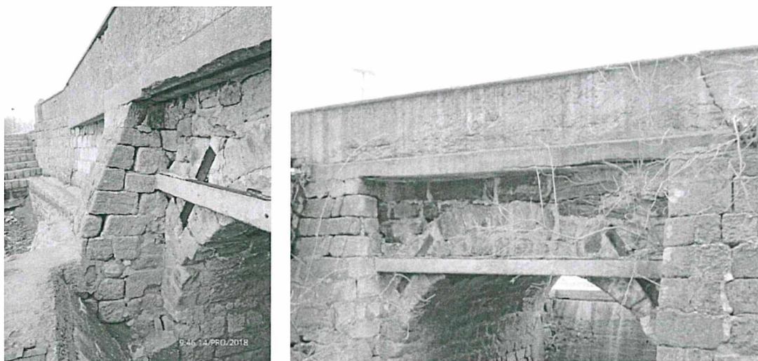
Obrázek 9 – Poškození čelních zdí na návodní (vlevo) a povodní (vpravo) straně mostu
